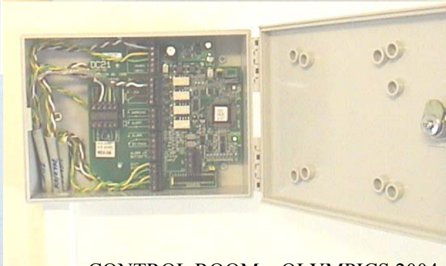
CONTROL ROOM – OLYMPICS 2004 ΛΙΜΑΝΙ ΗΡΑΚΛΕΙΟΥ
